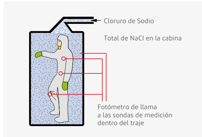
Imagen 2: Prueba de fuga interna en el traje
